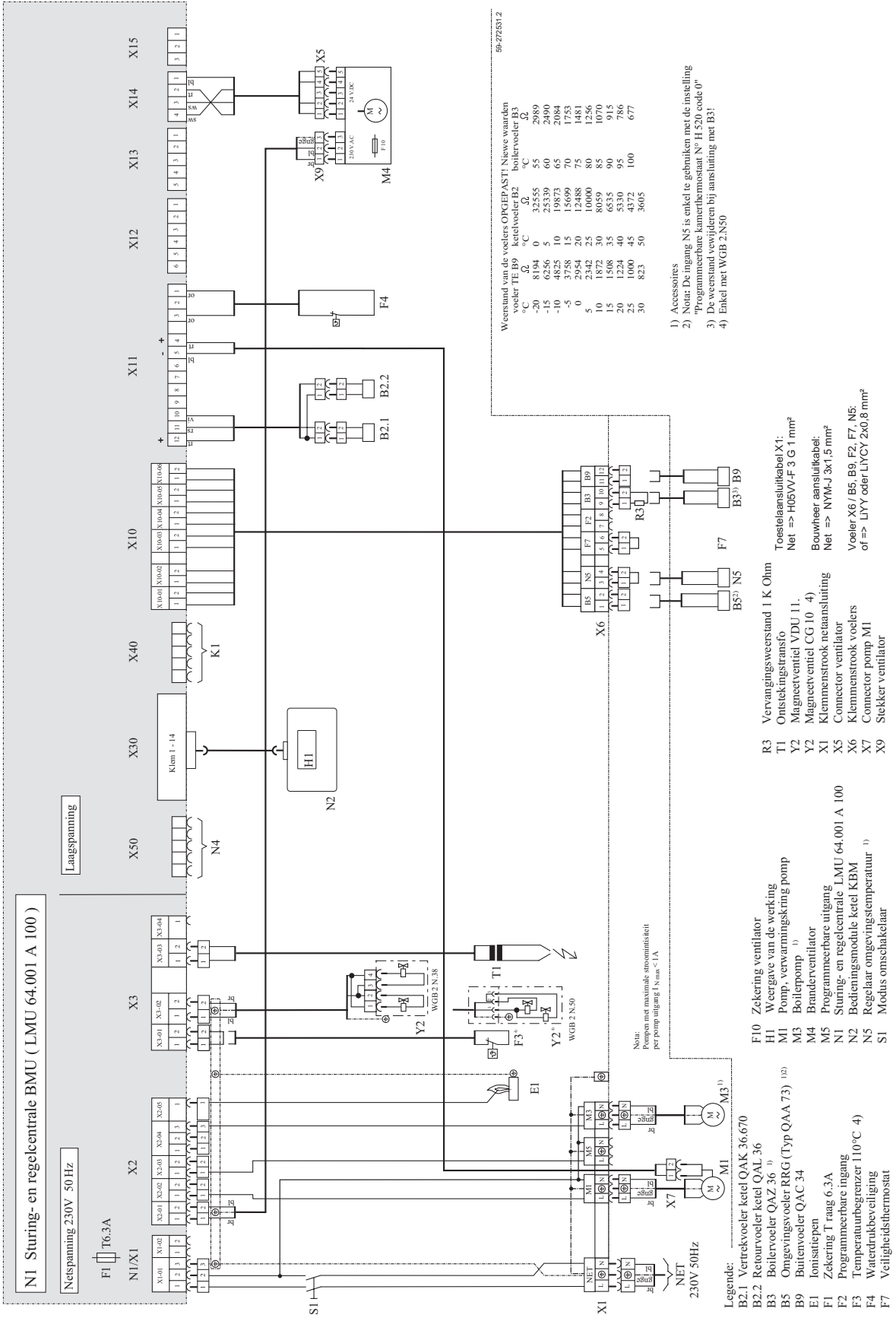
Schets 4 Bedradingsschema ketel
